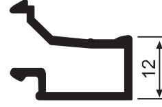
YS 5536 0,230 kg/m
