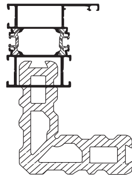
KT 122 YS 5543 Hazır Kesilmiş Köşe Takozu 18.5 mm
