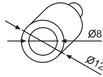
İspanyolek Pimi
