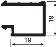
YS 344 0,245 kg/m
