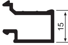
YS 5526 0,240 kg/m
