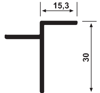
YS 5527 Kasa T'si 0,200 kg/m
