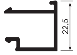
YS 5576 0,260 kg/m
