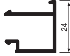
YS 5524 0,260 kg/m
