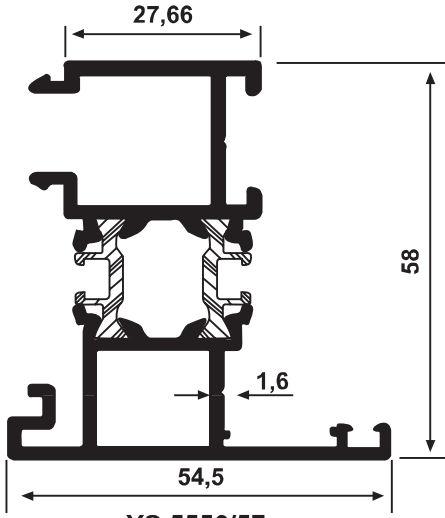
YS 5556/57 Çift Kapı Adaptörü 1,285 kg/m
