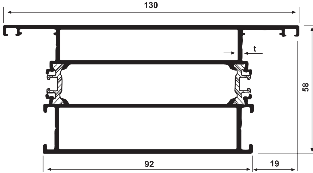
YS 5587/88 Geniş Orta Kayıt (t=2 mm) 2,820 kg/m
