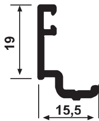
YS 5535 Kasa Tırnağı 0,165 kg/m
