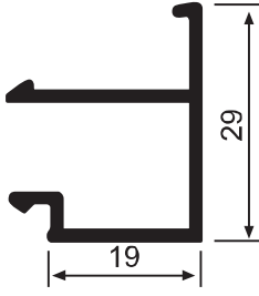
YS 5599 0,275 kg/m
