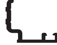
YS 5523 0,185 kg/m
