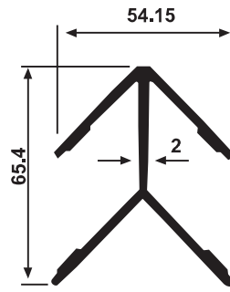
YG 4686 0,854 kg/m Sİ 58 Çavuş Bağlantı
