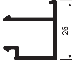
YS 397 0,265 kg/m
