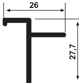
YS 1512 Kasa T'si 0,180 kg/m
