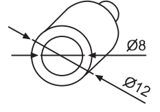
İspanyolet Pimi
