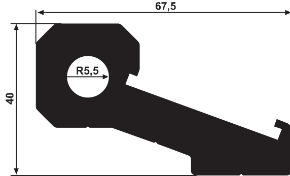
YG 1831 3,100 kg/m
