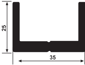
YS 4180 Dik Bağlantı 0,800 kg/m
