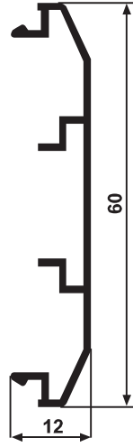
YG 4027 Çarpma Adaptörü 0,321 kg/m
