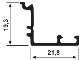
YS 4179 Ek Kulak 0,210 kg/m
