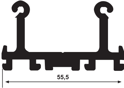
YG 4633 Dik Bağlantı 1,285 kg/m
