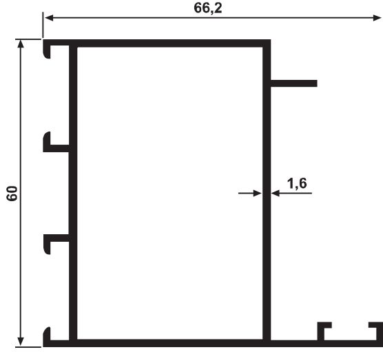
YG 4022 1,095 kg/m Kanat
