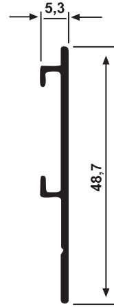
YS 1439 Pencere Adaptörü 0,225 kg/m
